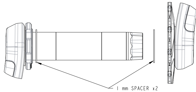
RF136 SPINDLE
